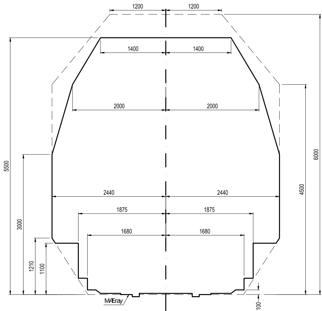
A.7 – Khổ giới hạn tiếp giáp kiến trúc trên đường thẳng trong cầu (Khổ đường 1435 mm)
