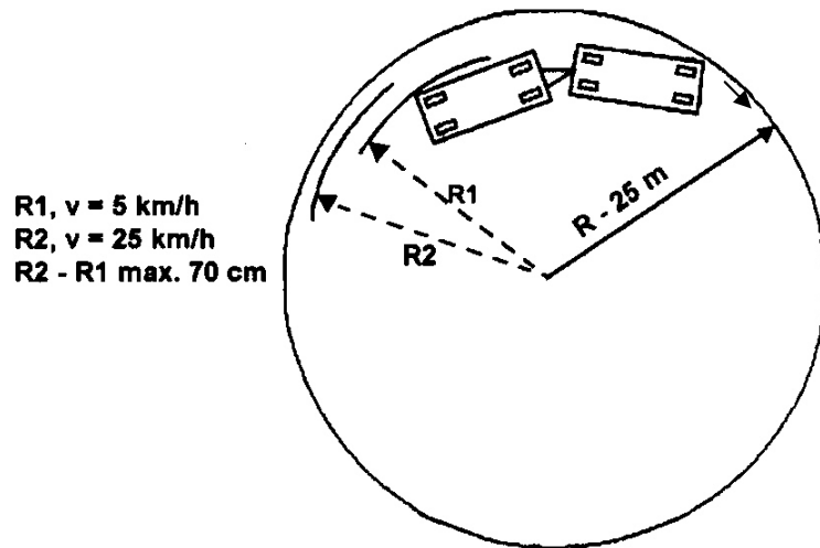
Hình 8: Quay vòng của xe ô tô kéo rơ moóc
