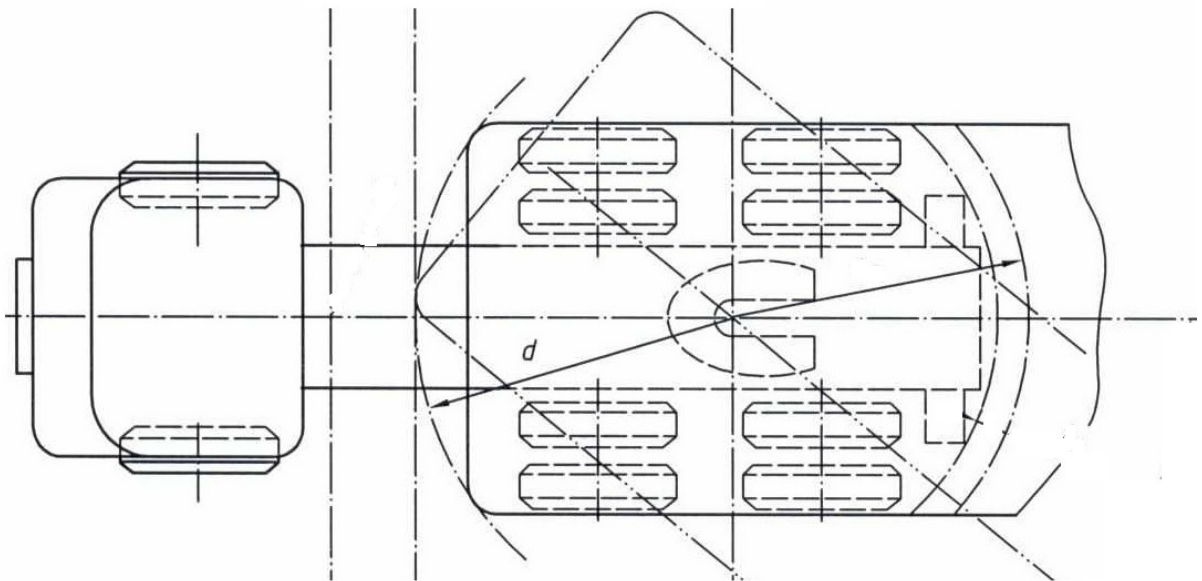
Hình 5: Bán kính khoảng sáng quay đầu phía trước của sơ mi rơ moóc
