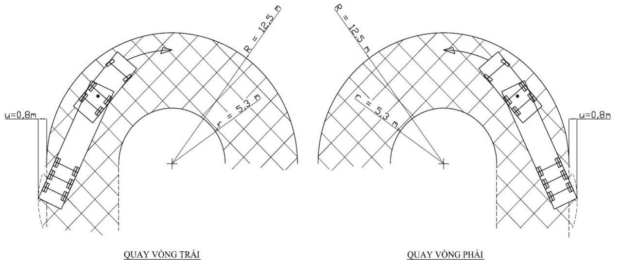
Hình 7: Quay vòng của đoàn xe kéo sơ mi rơ moóc
