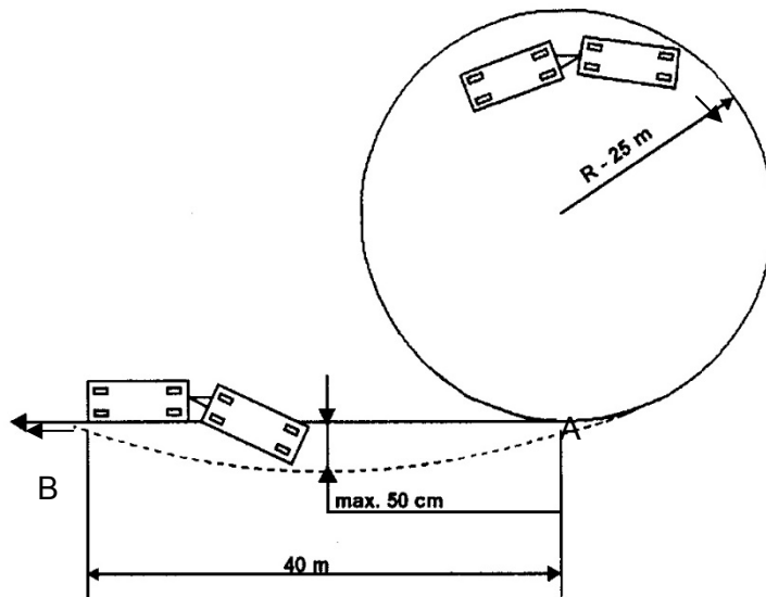
Hình 9: Quay vòng của xe ô tô kéo rơ moóc
