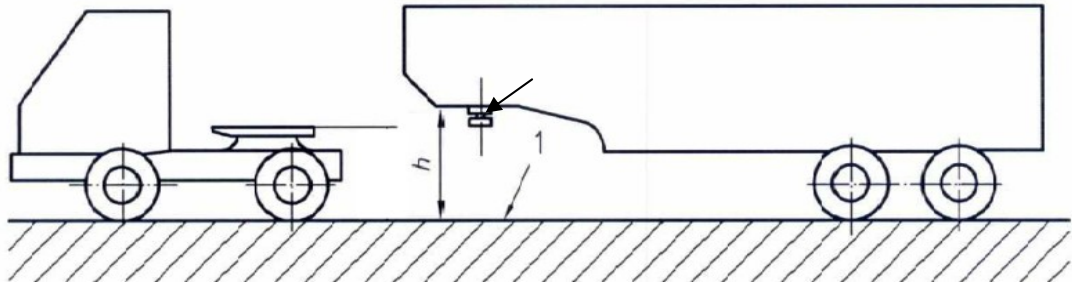
Hình 4: Chiều cao mặt tì lên mâm kéo của chốt kéo
