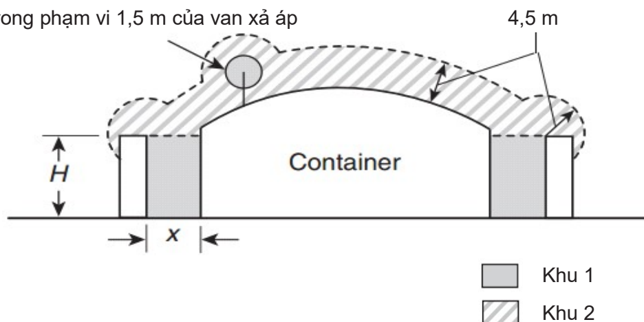
Hình 1 (b) - Chiều cao đê lớn hơn khoảng cách từ container đến đê ( H > x )
