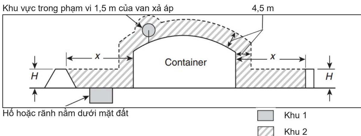
Hình 1 (a) - Chiều cao đê nhỏ hơn khoảng cách từ bồn chứa đến đê ( H < x )
