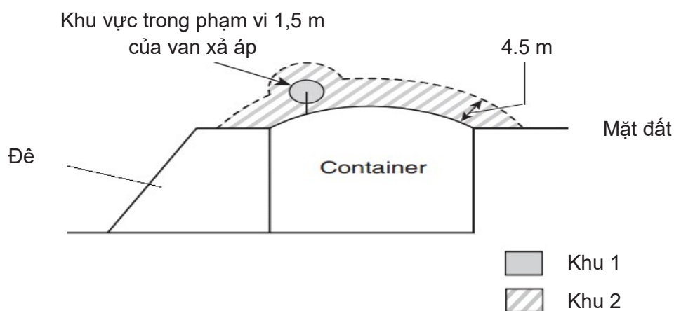
Hình 1 (c) Bình chứa có mức chất lỏng dưới lớp phân loại bên dưới đỉnh đê
