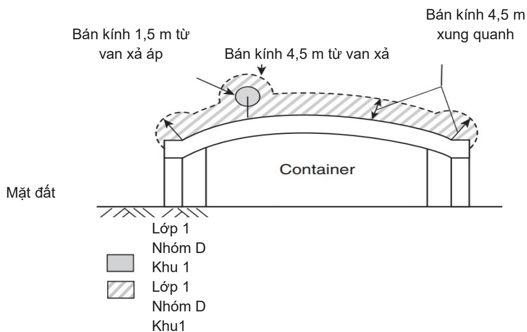
Hình 1 (d) - Hệ thống bồn chứa hỗn hợp và bồn chứa màng
